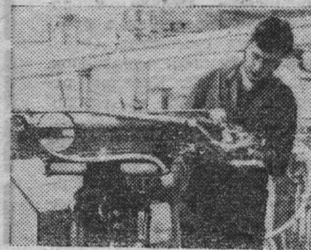
ВНР. Промышленные работы, заменяющие людей в трудоемких операциях, связанных с производством телевизионных кинескопов, выпускает завод в Дендьеше. Это предприятие является филиалом венгерского электротехнического объединения «Эдешюльт иззо», изделия которого известны под маркой «Тунгграм». Новый вид продукции — роботы — экспортируется в Советский Союз.
