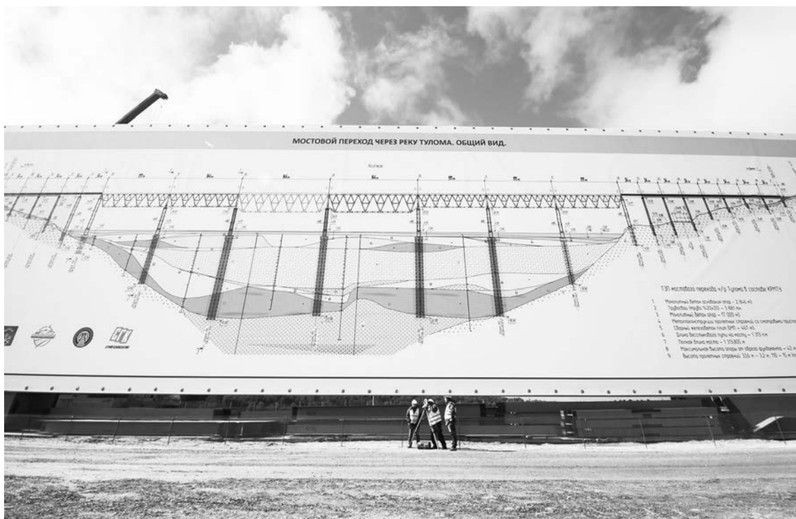
Железнодорожный мост через реку Тулому спроектирован с учетом сложной геологии и рельефа на обоих берегах.
