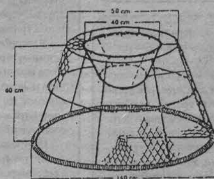
СХЕМА КРАБОВОЙ ЛОВУШКИ
